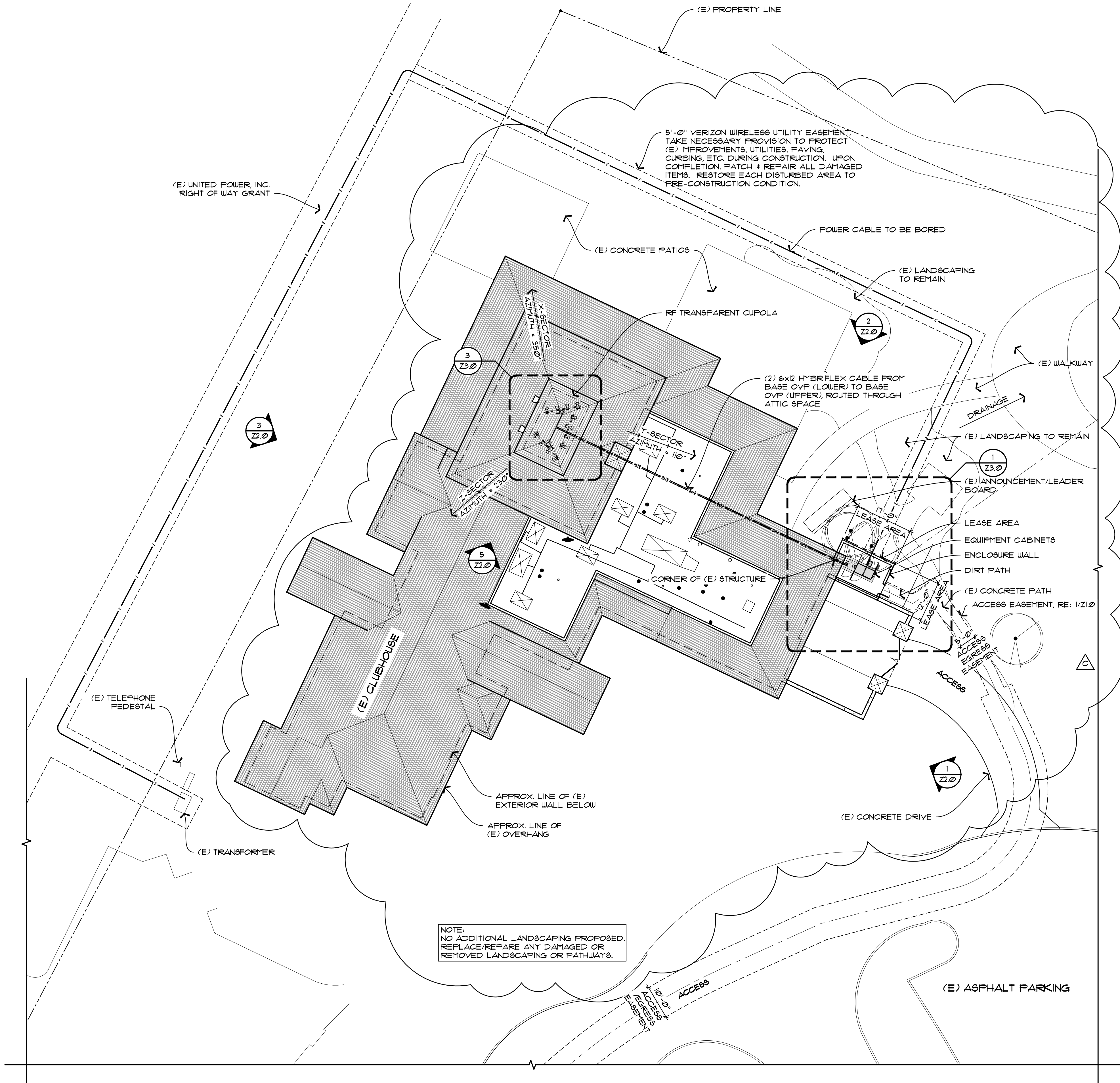
1 Z1.1 ENLARGED SITE PLAN SCALE: 1/16" = 1'-0" RE: 1/Z1
